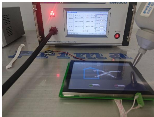
图 4-2 ESD 测试图
