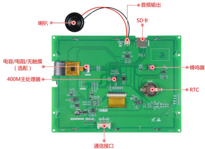
图 1-4 硬件配置图
